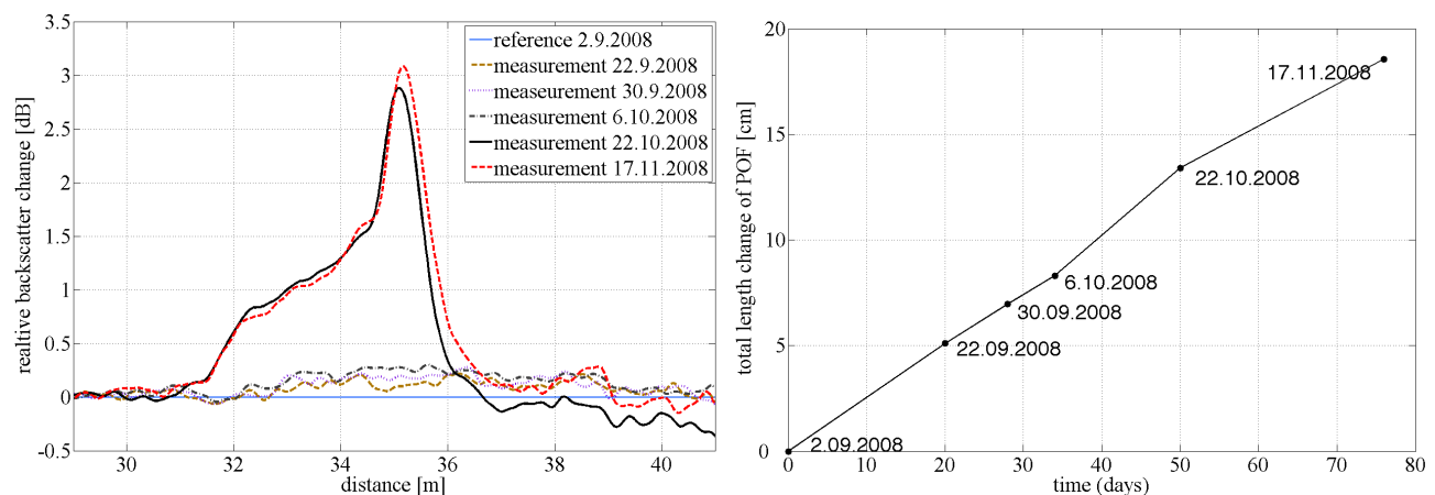
Rys.5 Wyniki pomiarów metodą POF OTDR.
